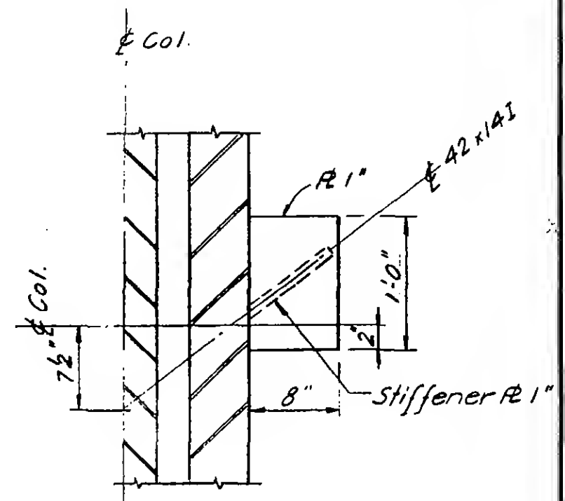
Section d-d
