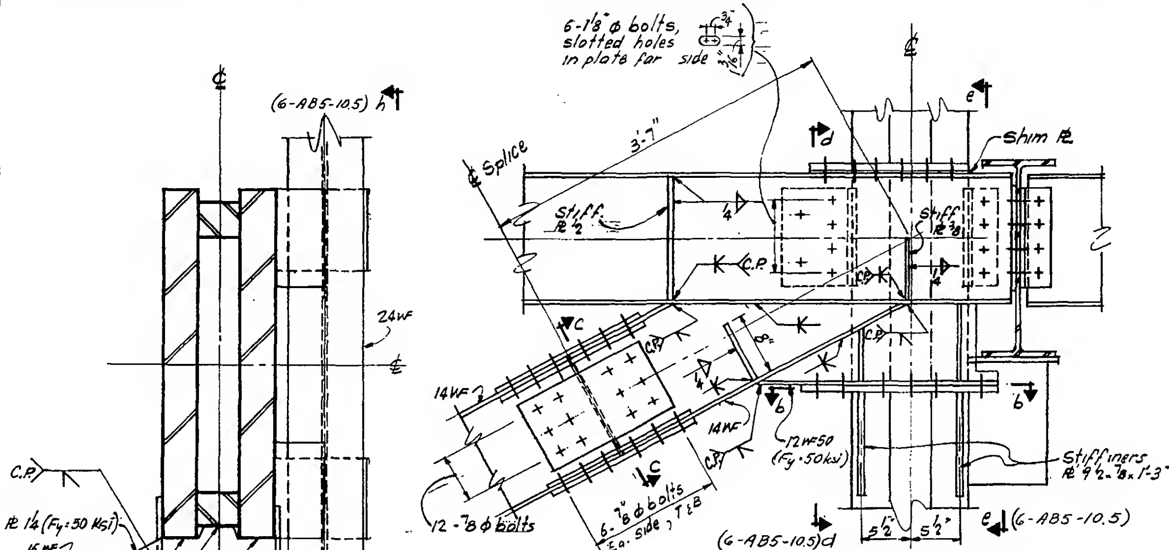
SECTION a-a
