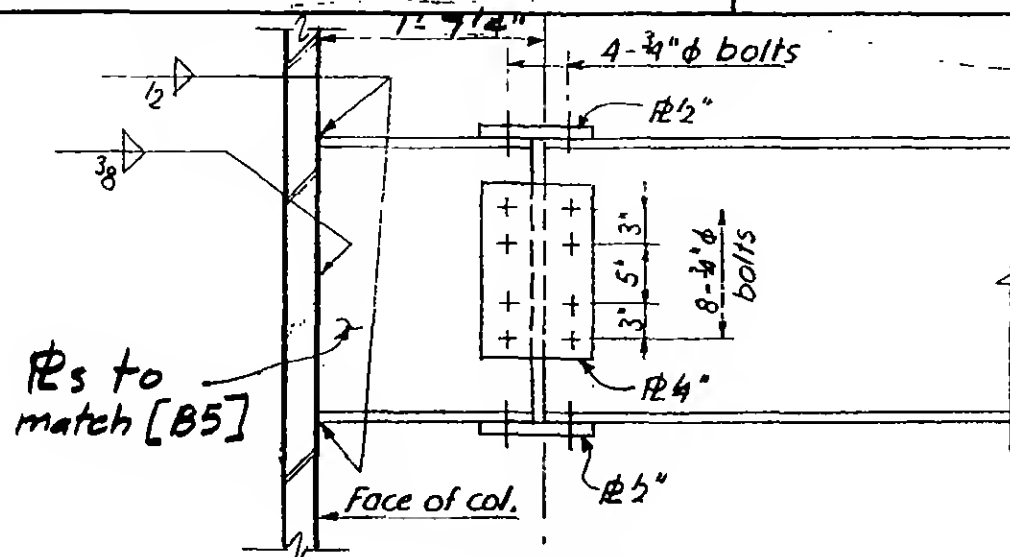
Section a-a - E3
