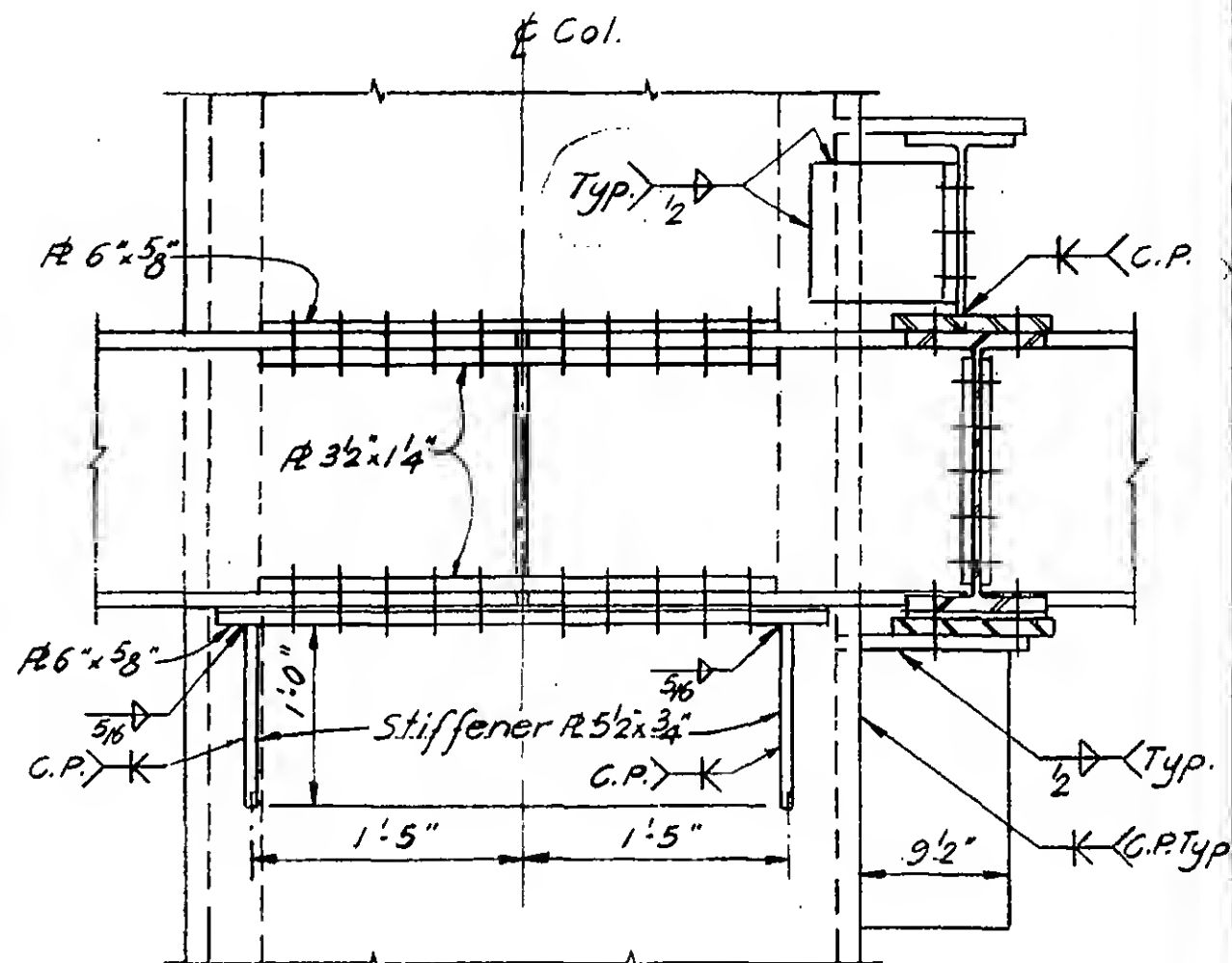
Elevation a-a
