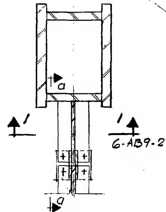
Plan E3
