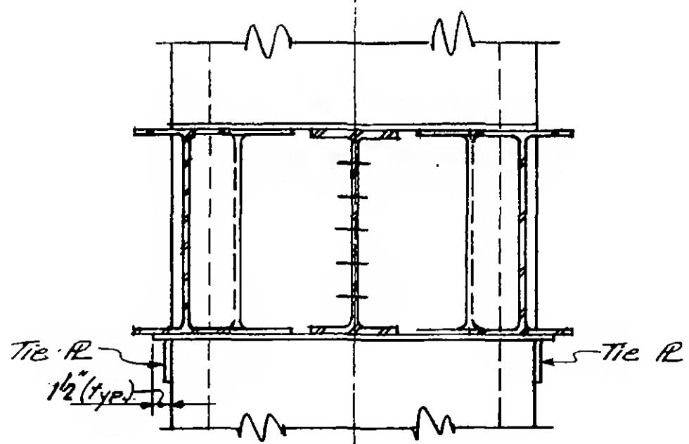
Section d-d
