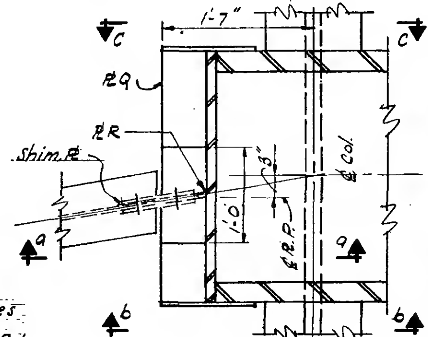
Det. 851 F
