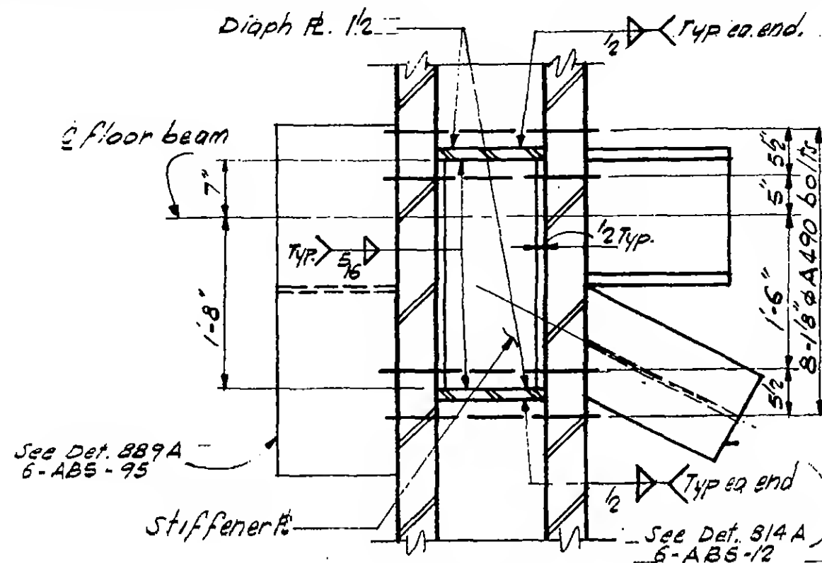
Section a-a
