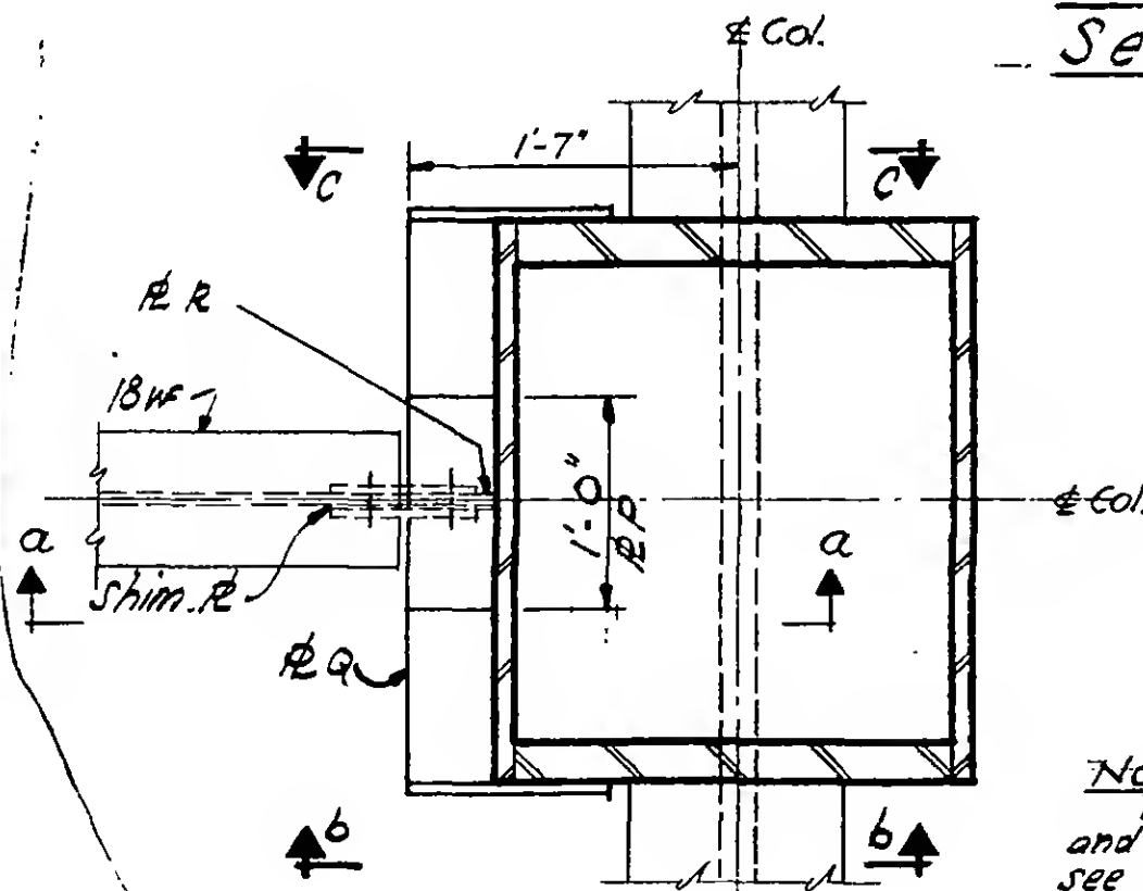
Det. 851 A, B, & E
