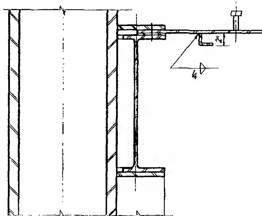
Section a-a
