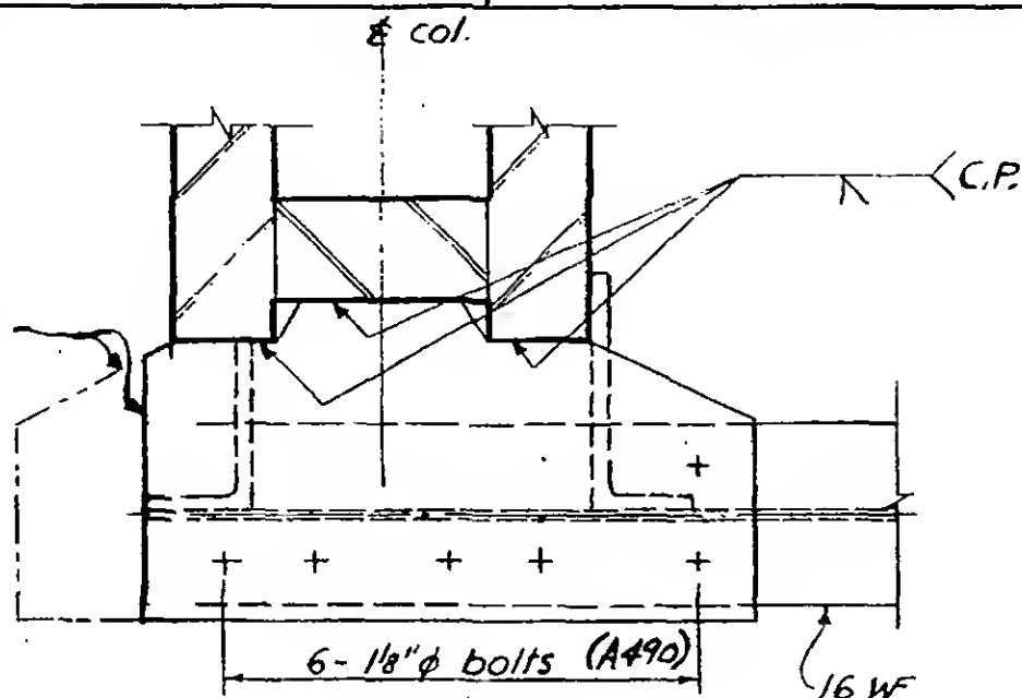
Section d-d
