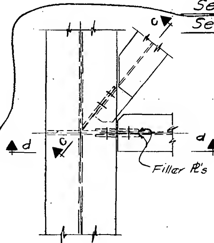
Plan Det. 846 B
