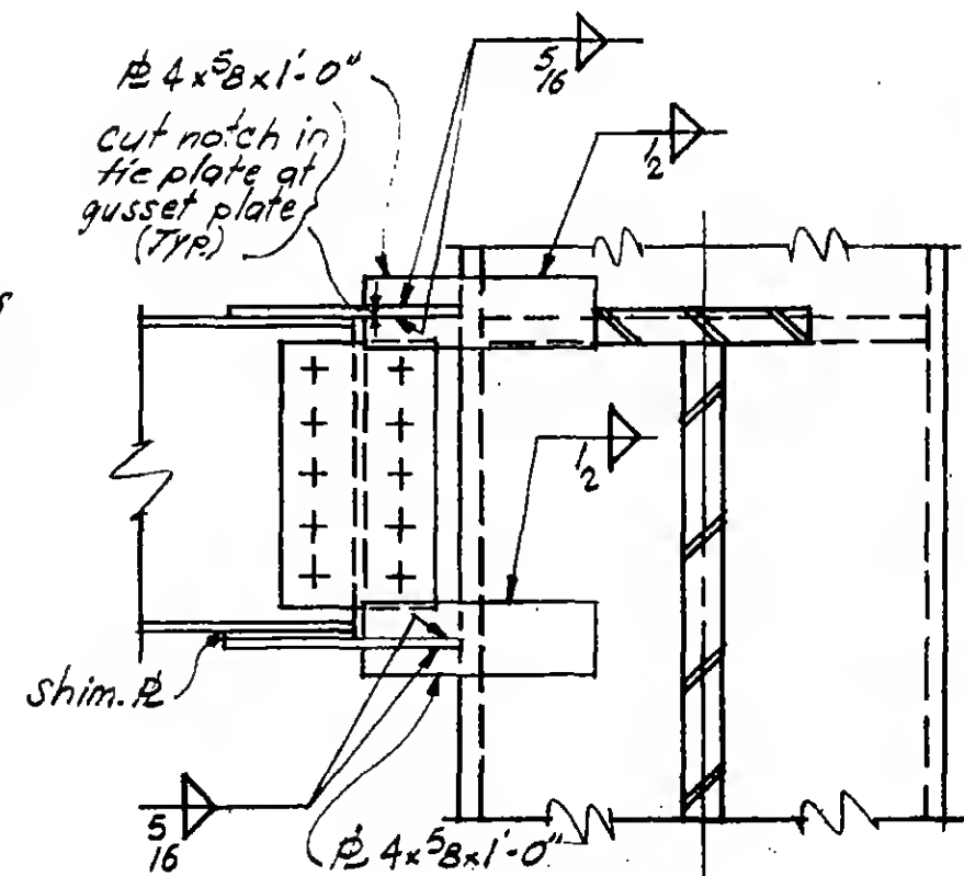
Section d-d
