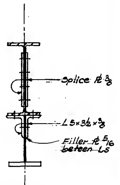
Section d-d
