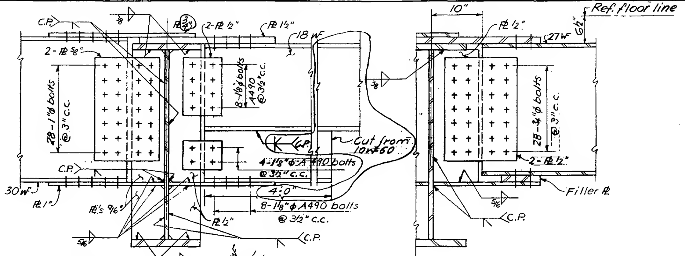
Section a-a
