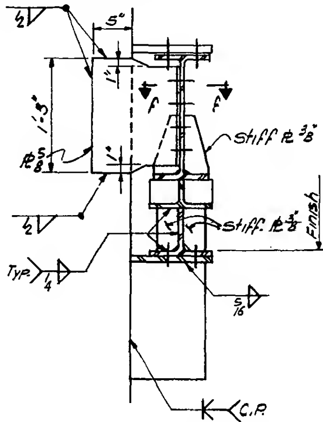
SECTION d-d
