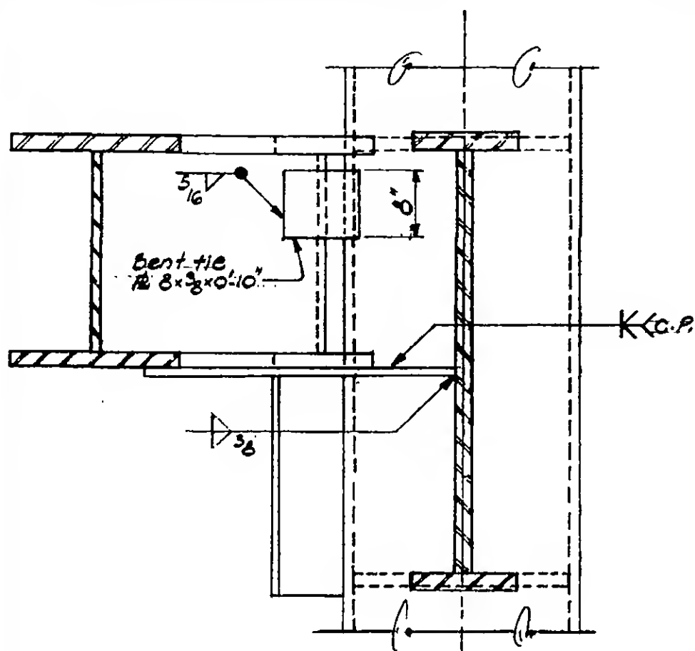
Section d-d
