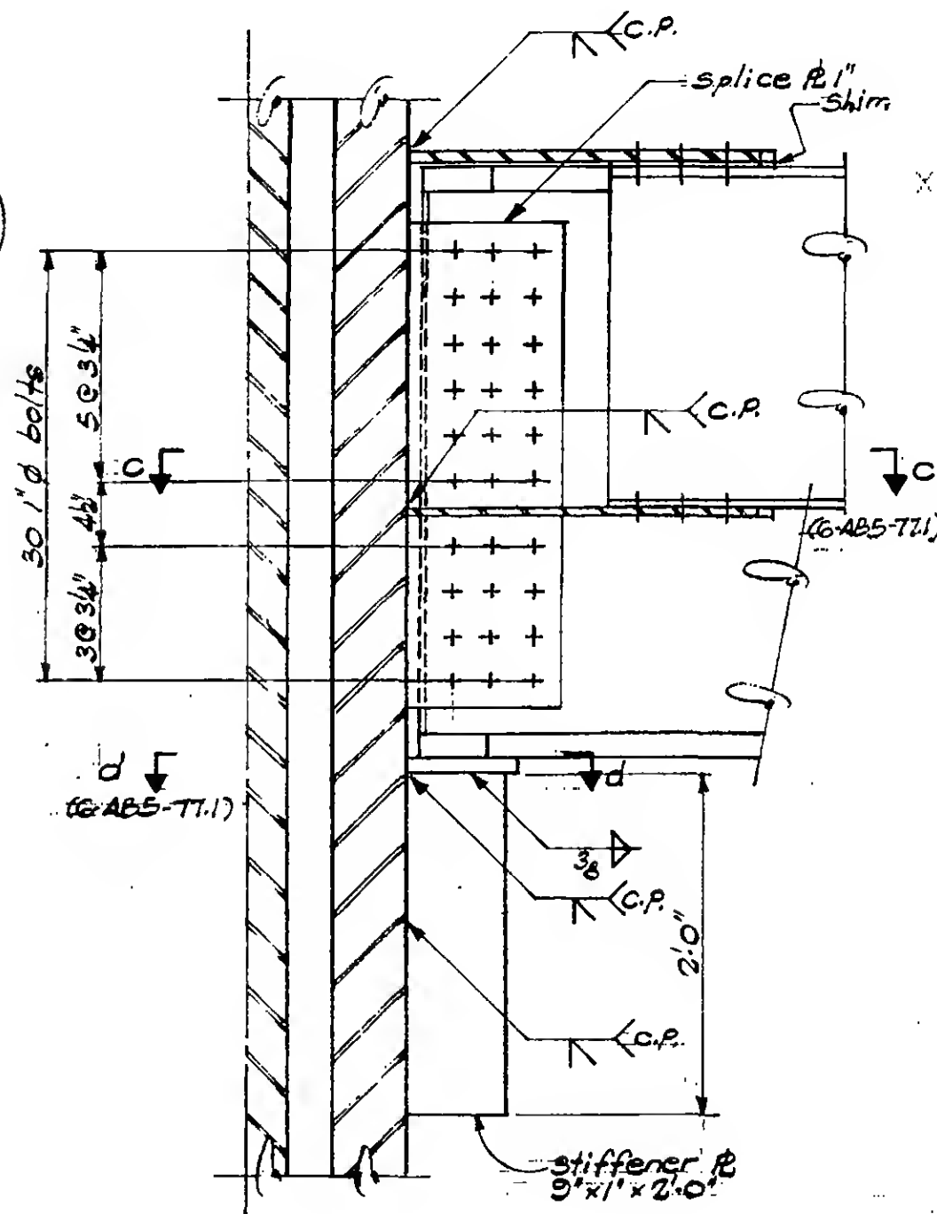
Section a-a
