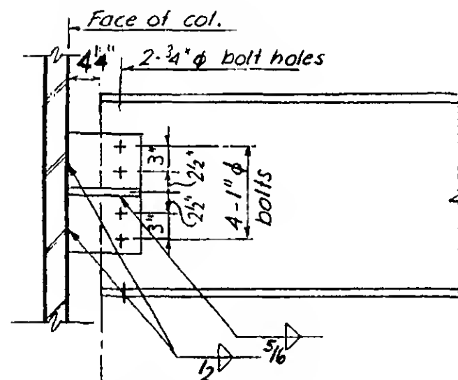
Section a-a - E2
